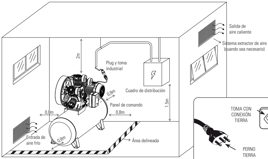
FIGURA 7.10 DETALLE DE LA ALIMENTACIÓN ELÉCTRICA E INSTALACIÓN DEL COMPRESOR A PARTIR DEL CUADRO DE DISTRIBUCIÓN (CD)
