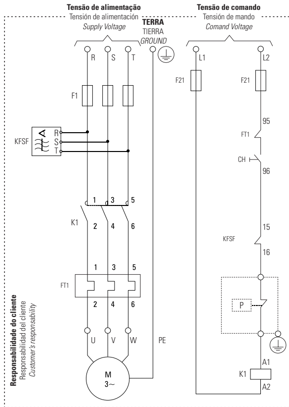
4 MOTORES TRIFÁSICOS - PARTIDA DIRETA MOTORES TRIFÁSICOS - PARTIDA DIRETA THREE-PHASE MOTOR WITH DIRECT STARTER
