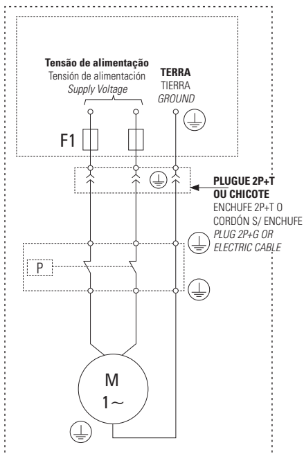
1 ESQUEMA DE CONEXÃO ELÉTRICA MONOFÁSICA (MOTOR ESPECIAL C/ PROTETOR TÉRMICO) ESQUEMA DE CONEXIÓN ELÉCTRICA MONOFÁSICA (MOTOR ESPECIAL CON PROTECTOR TÉRMICO) ELECTRICAL CONNECTION DIAGRAM (SPECIAL MOTOR WITH THERMAL PROTECTOR)
