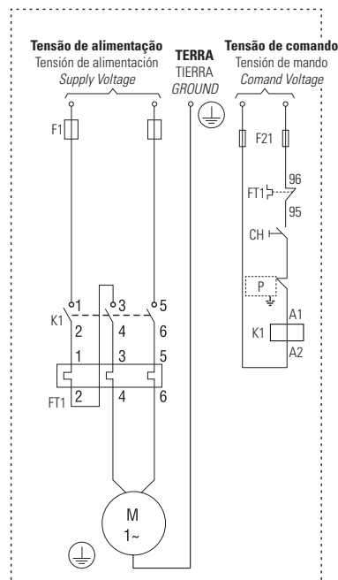
2 ESQUEMA DE CONEXÃO ELÉTRICA MONOFÁSICA (MOTOR STANDARD) ESQUEMA DE CONEXIÓN ELÉCTRICA MONOFÁSICA (MOTOR STANDARD) ELECTRICAL CONNECTION DIAGRAM (STANDARD MOTOR)
