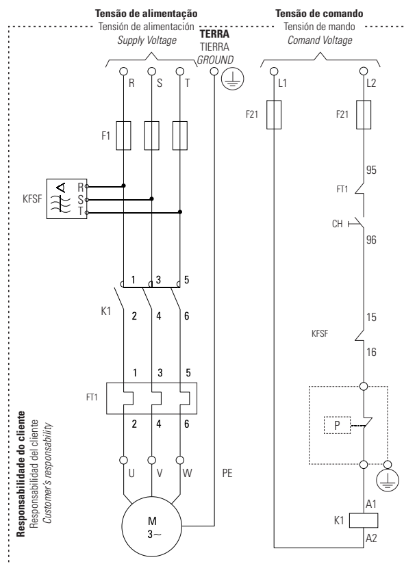
4 MOTORES TRIFÁSICOS - PARTIDA DIRETA MOTORES TRIFÁSICOS - PARTIDA DIRECTA THREE-PHASE MOTOR WITH DIRECT STARTER
