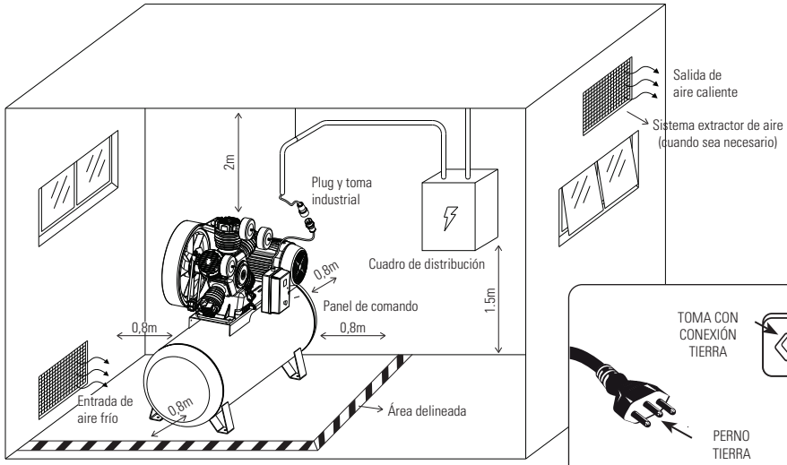
FIGURA 7.10 DETALLE DE LA ALIMENTACIÓN ELÉCTRICA E INSTALACIÓN DEL COMPRESOR A PARTIR DEL CUADRO DE DISTRIBUCIÓN (CD)
